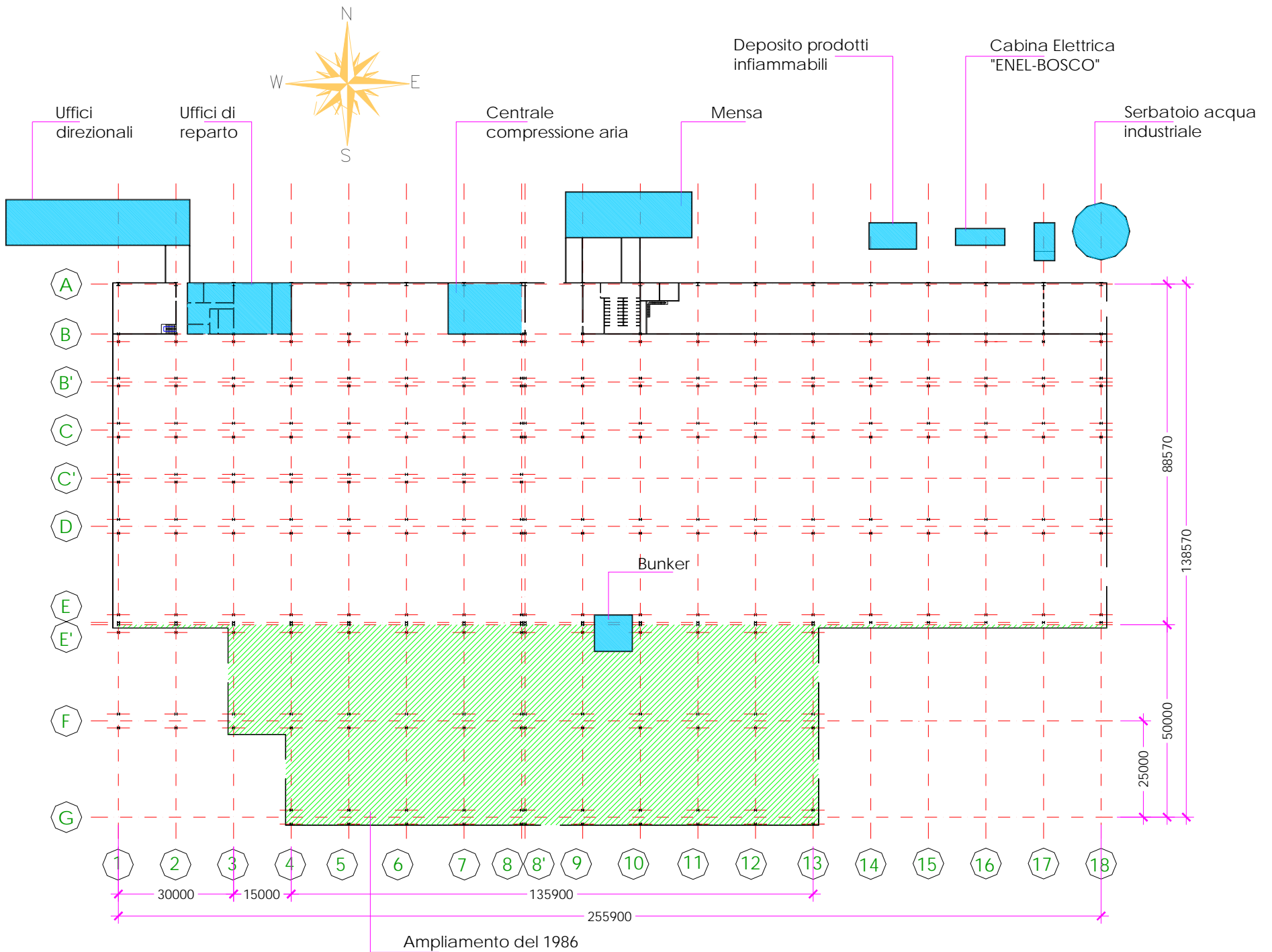
PLANIMETRIA GENERALE
